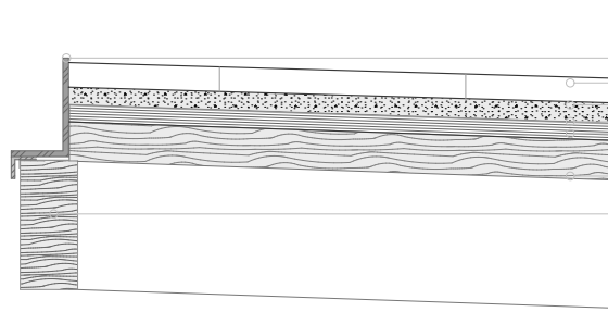
Detalle cubierta 1:10
