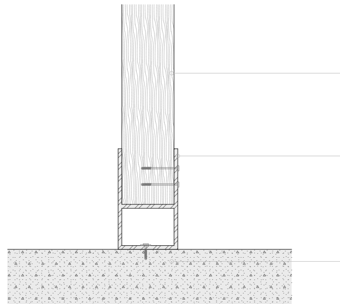
Unión columna-piso 1:10
