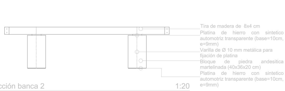
Sección banca 2 1:20
