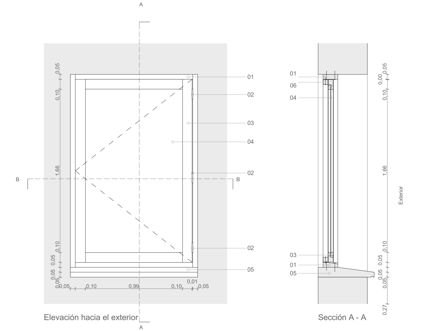
Ventana movil batiente hacia el exterior
