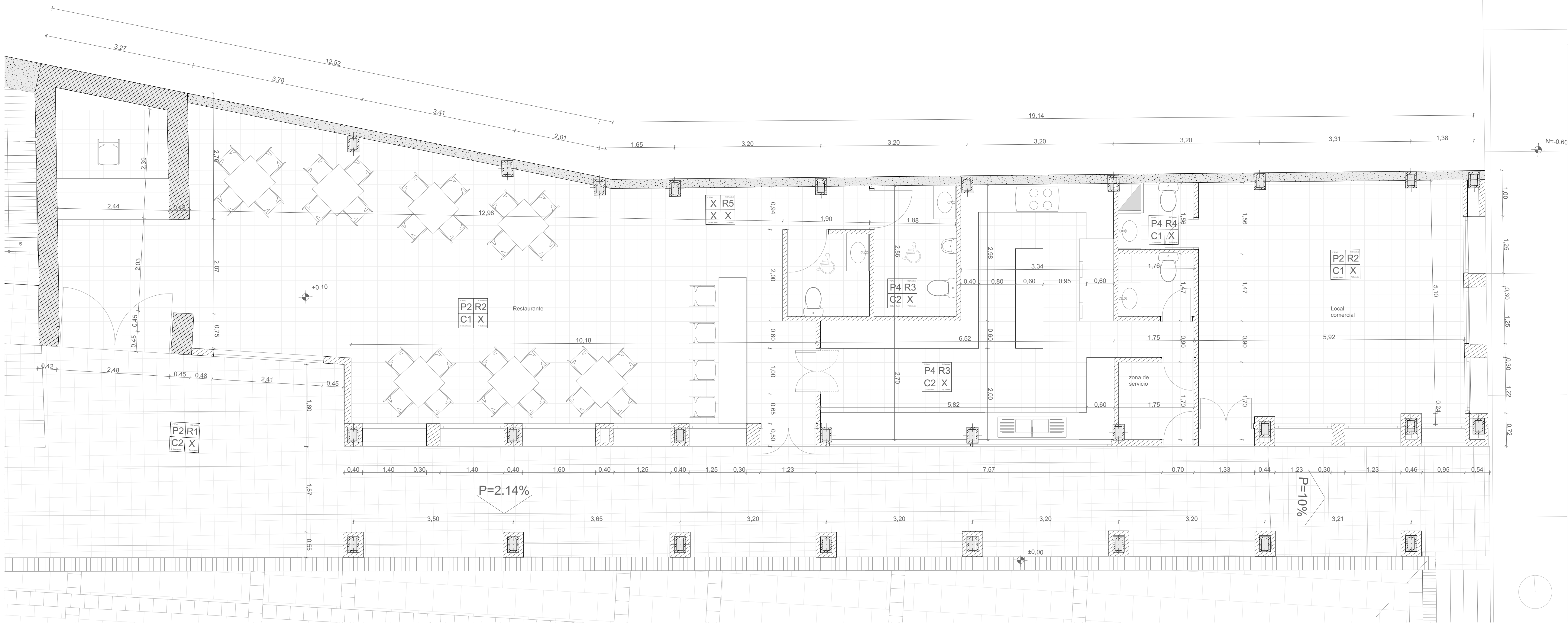
Planta baja (edificio Huayna Capac)
