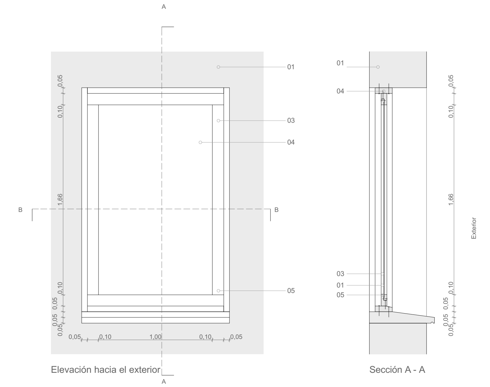
Ventana fija
