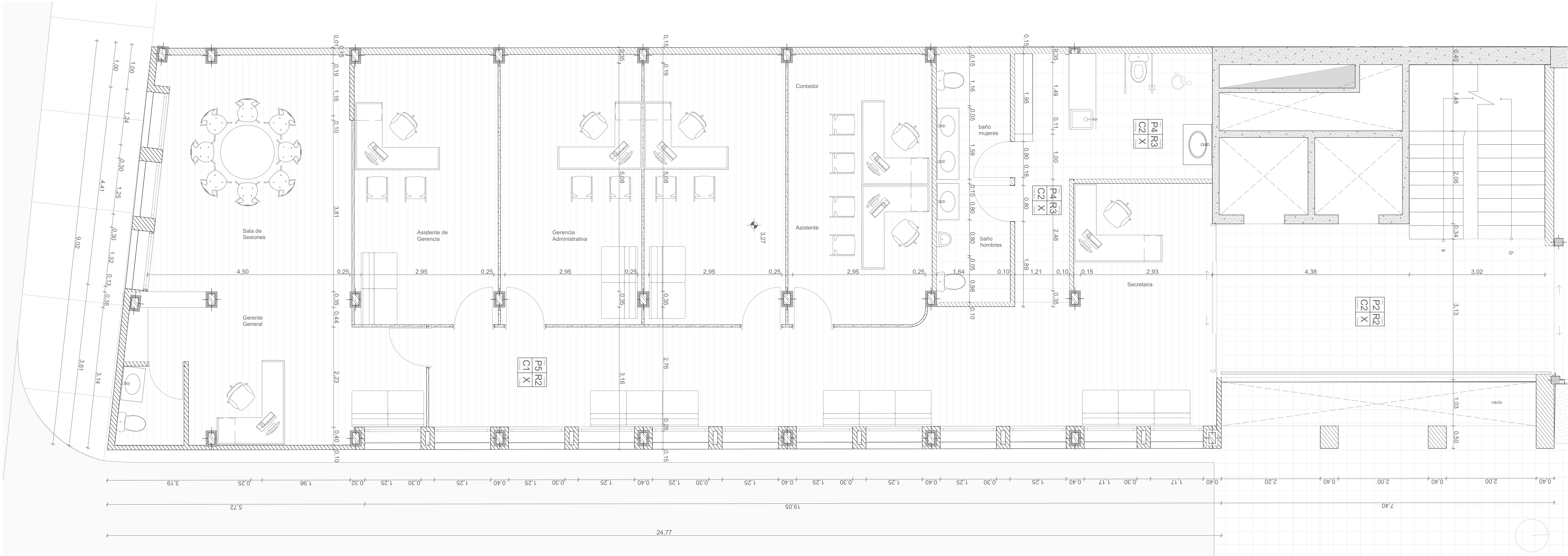
Planta alta (edificio Bolívar)
