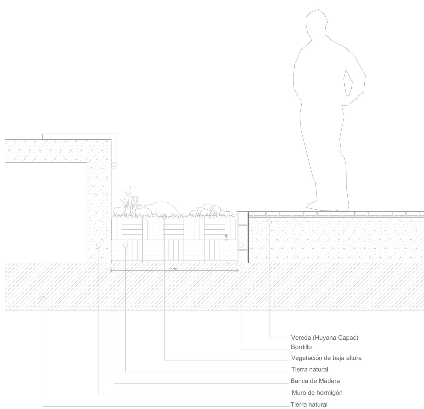
Sección detalle jardinera (Huayna Capac) esc:1_20
