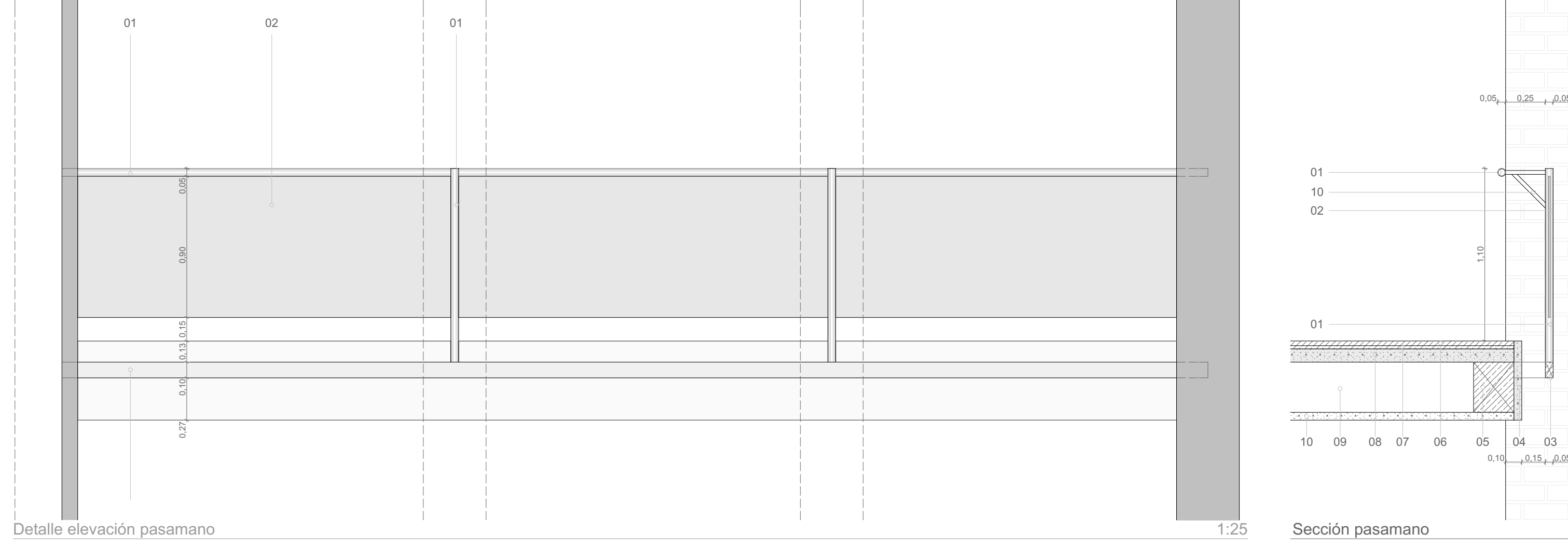
Detalle elevación pasamano 1:25
