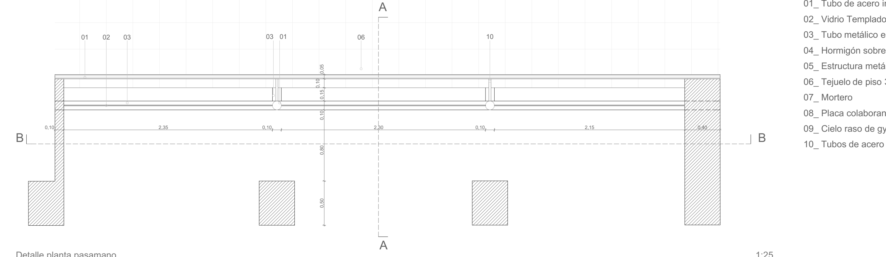
Detalle planta pasamano 1:25
