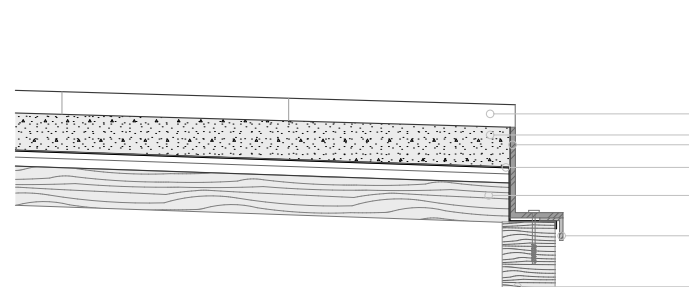
Detalle cubierta 2 1:10
