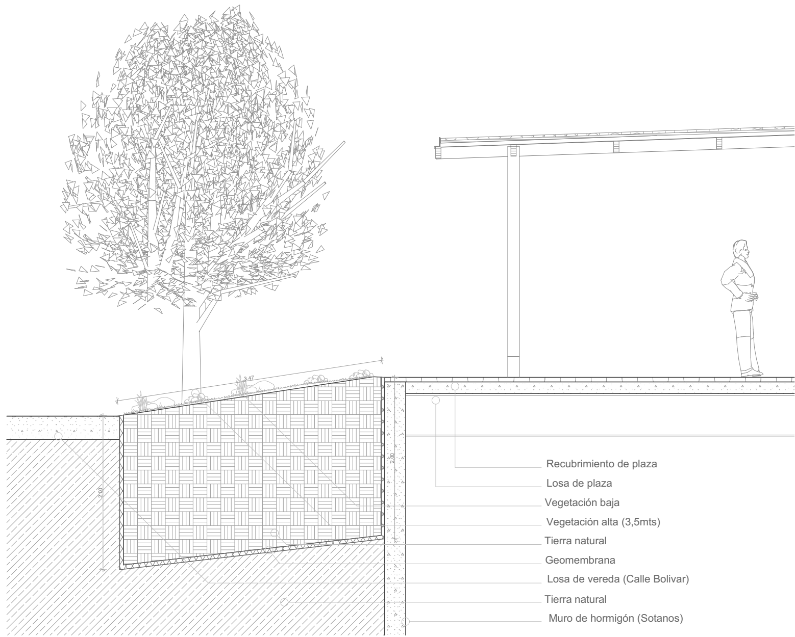
D01 Detalle sección jardinera (calle Bolivar) 1:50
