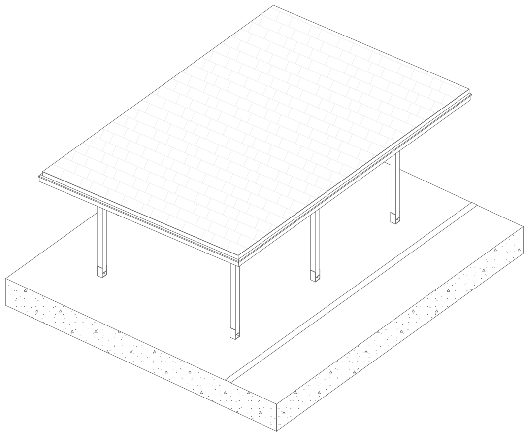
Tejuelo de 30x30x2,5 cm, perfil metálico L
