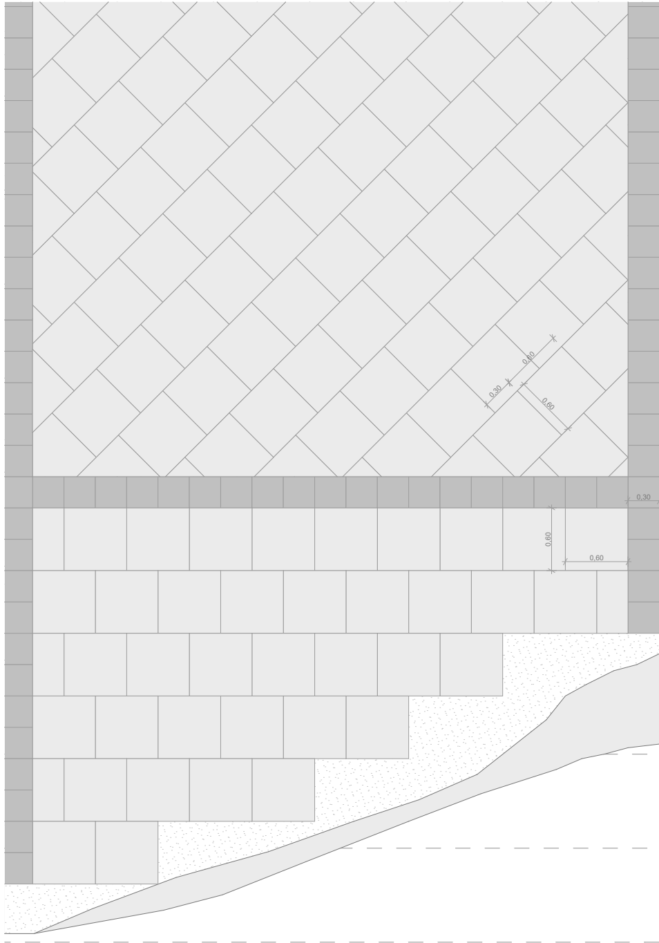
Planta de detalle piso 1:50
