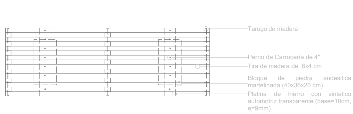
Planta banca 2 1:20
