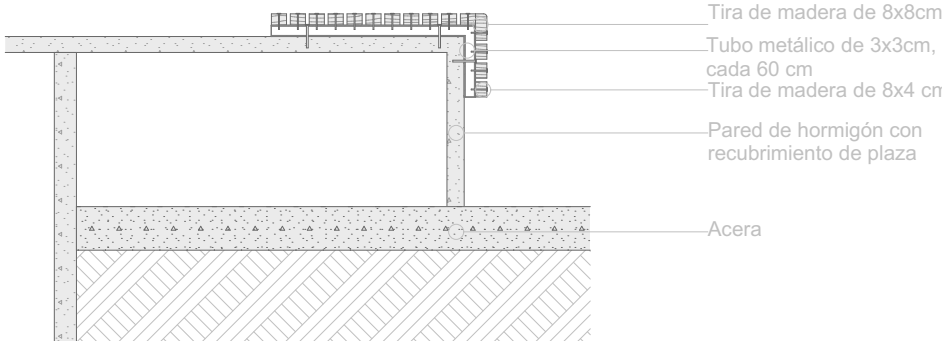
Sección banca 1 1:20
