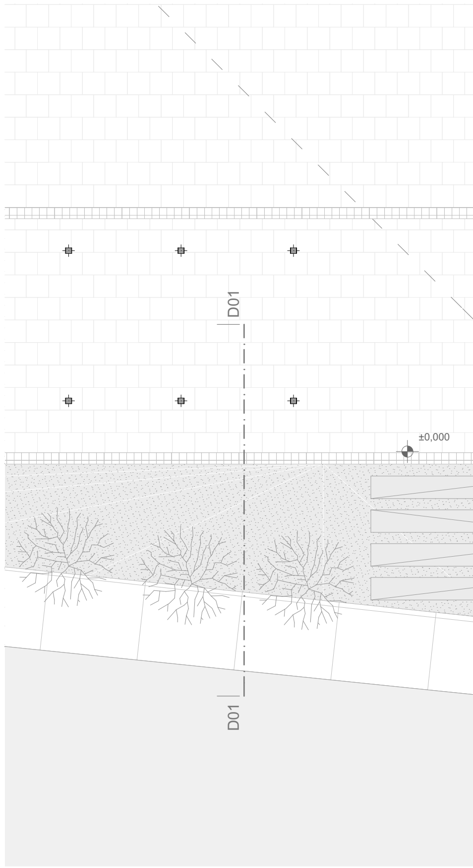
Detalle planta jardinera (calle Bolivar) 1:100
