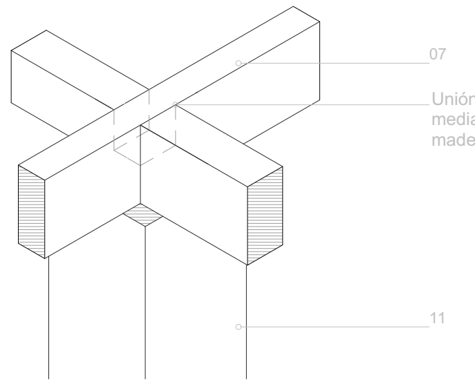
Unión vigas 1:20
