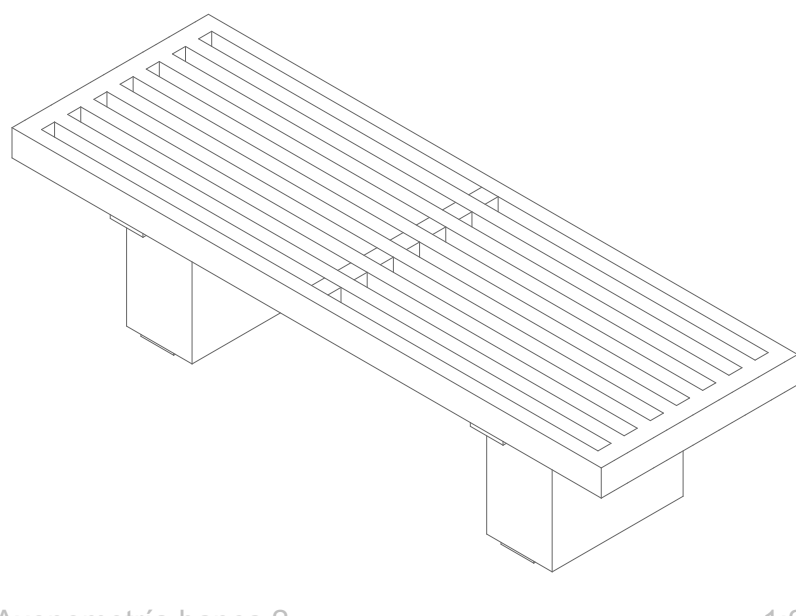
Axonometría banca 2 1:20
