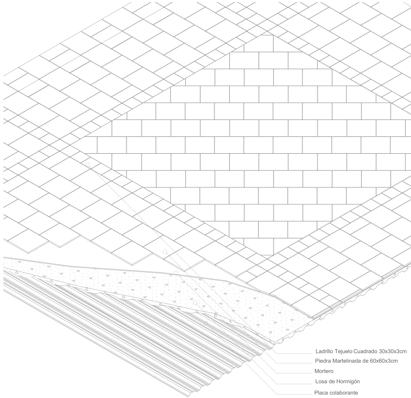
Axonometría detalle piso 1:50
