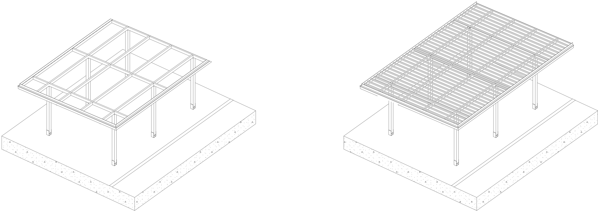
Base de columnas metálicas, Columnas de 15x15cm de romerillo, Vigas de 7x14cm romerillo con unión a media madera
