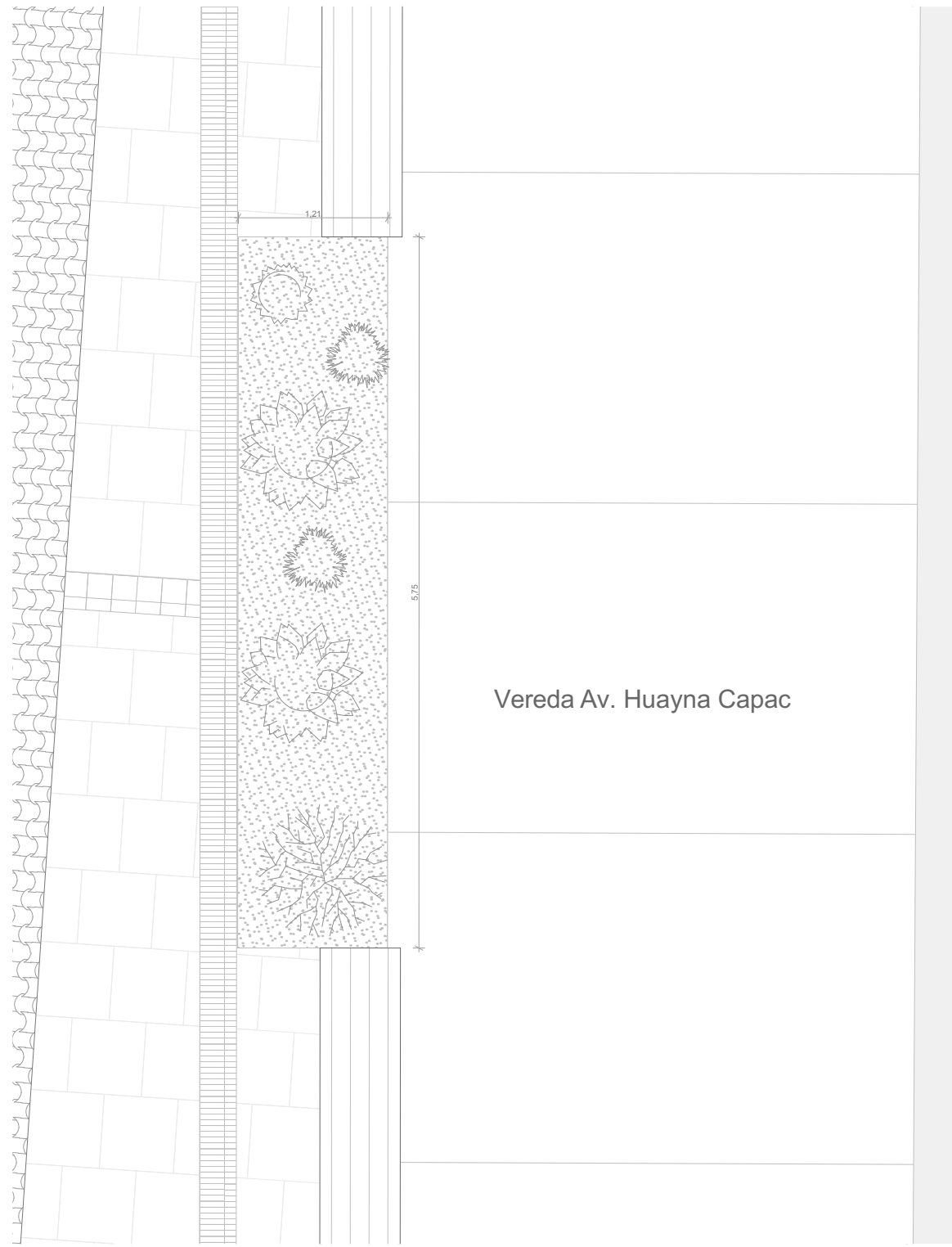
Detalle planta jardinera (Huayna Capac) 1:50
