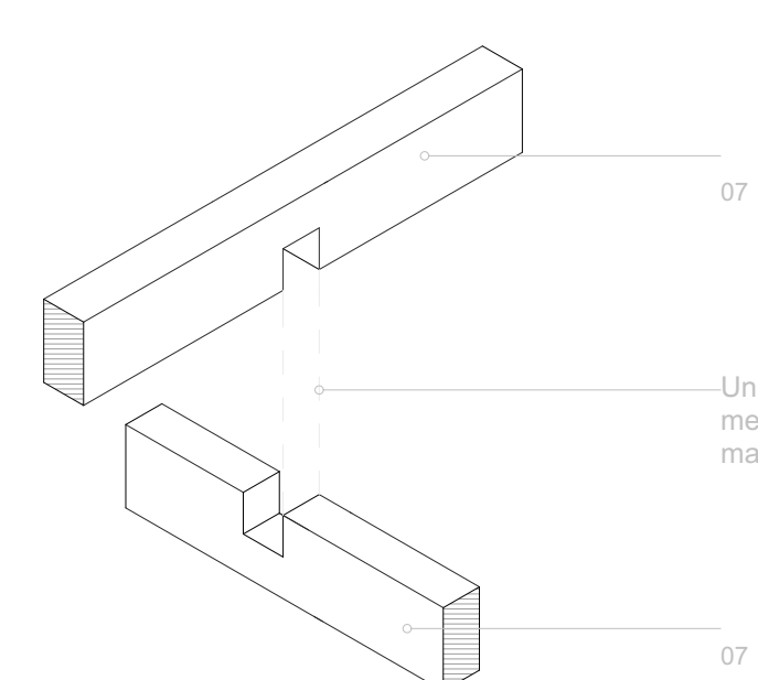
Unión vigas 1:20
