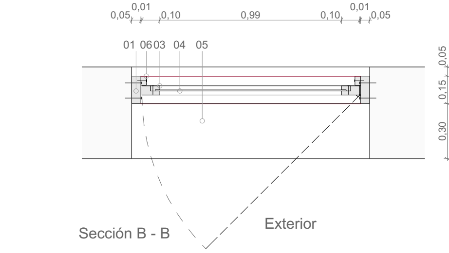
deetalles de ventaneria (2) 1:20
