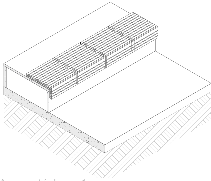
Axonometría banca 1
