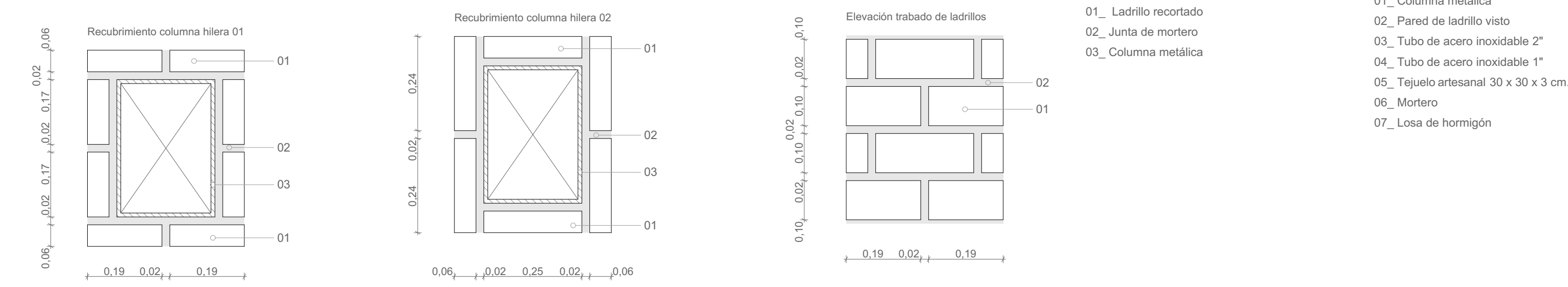
deetalles de ventaneria (2) 1:20
