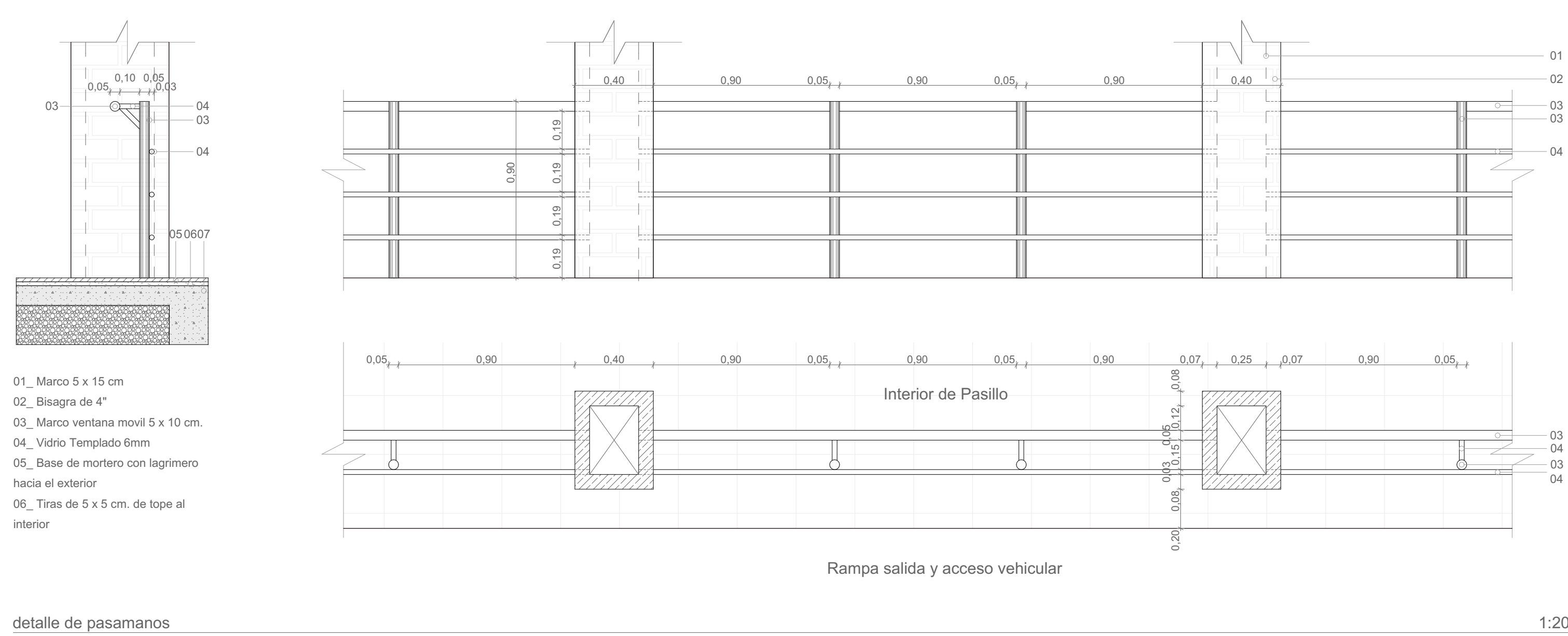
detalle de pasamanos 1:20
