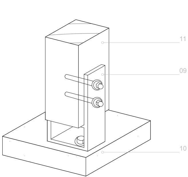
Unión columna-piso
